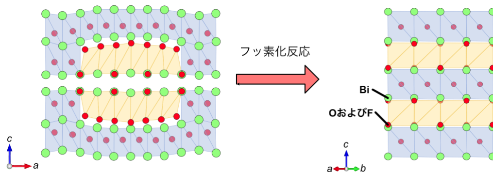
図 3: フッ素化反応前後での Bi-O(-F) 層の構造変化の模式図。フッ素挿入により、 c 軸方向に蛍石ユニット（水色）と岩塩ユニット（オレンジ）が交互に積層する構造に変化しています。また、フッ素化により波のような構造の歪みが消失して、Bi-O(-F) 層が面内（ ab 方向）に平らになっています。
