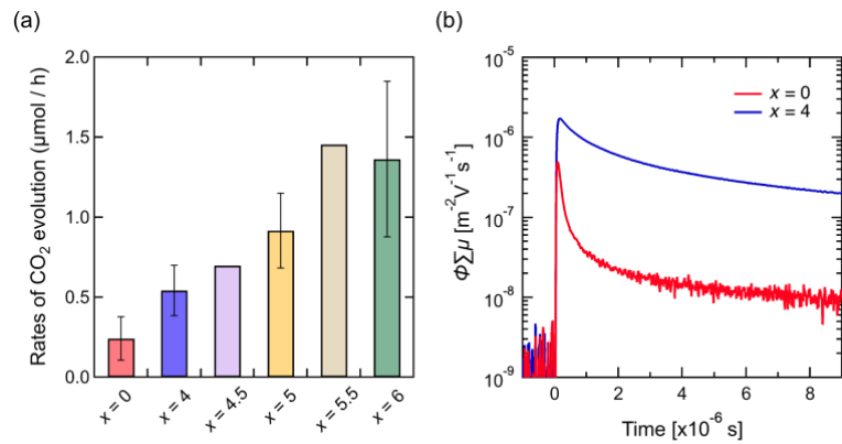
図 4: (a) 酢酸分解に対する光触媒活性。Bi 12 O 17-0.5x F x Cl 2 のフッ素量 x が増えるに従って、光触媒活性が大幅に向上しています。(b) フッ素化前後の光伝導度。フッ素化後に光伝導度の向上が見られ、光吸収によって生じた電子がスムーズに表面に移動することで、光触媒活性が向上したと考えられます。
