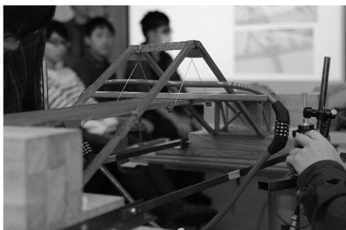
図4 構造力学・水理学実験第一 (ブリッジコンペティション)
